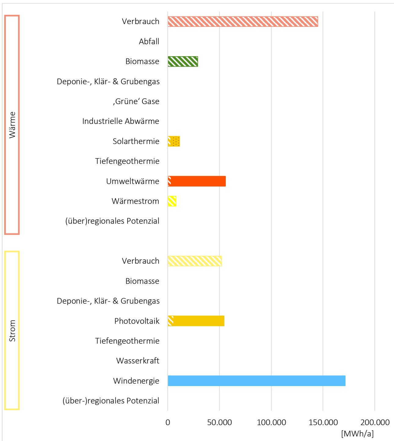
Abbildung 25: Potenzialübersicht erneuerbare Energien (Summe aus Bestand und zusätzlichem Potenzial)
