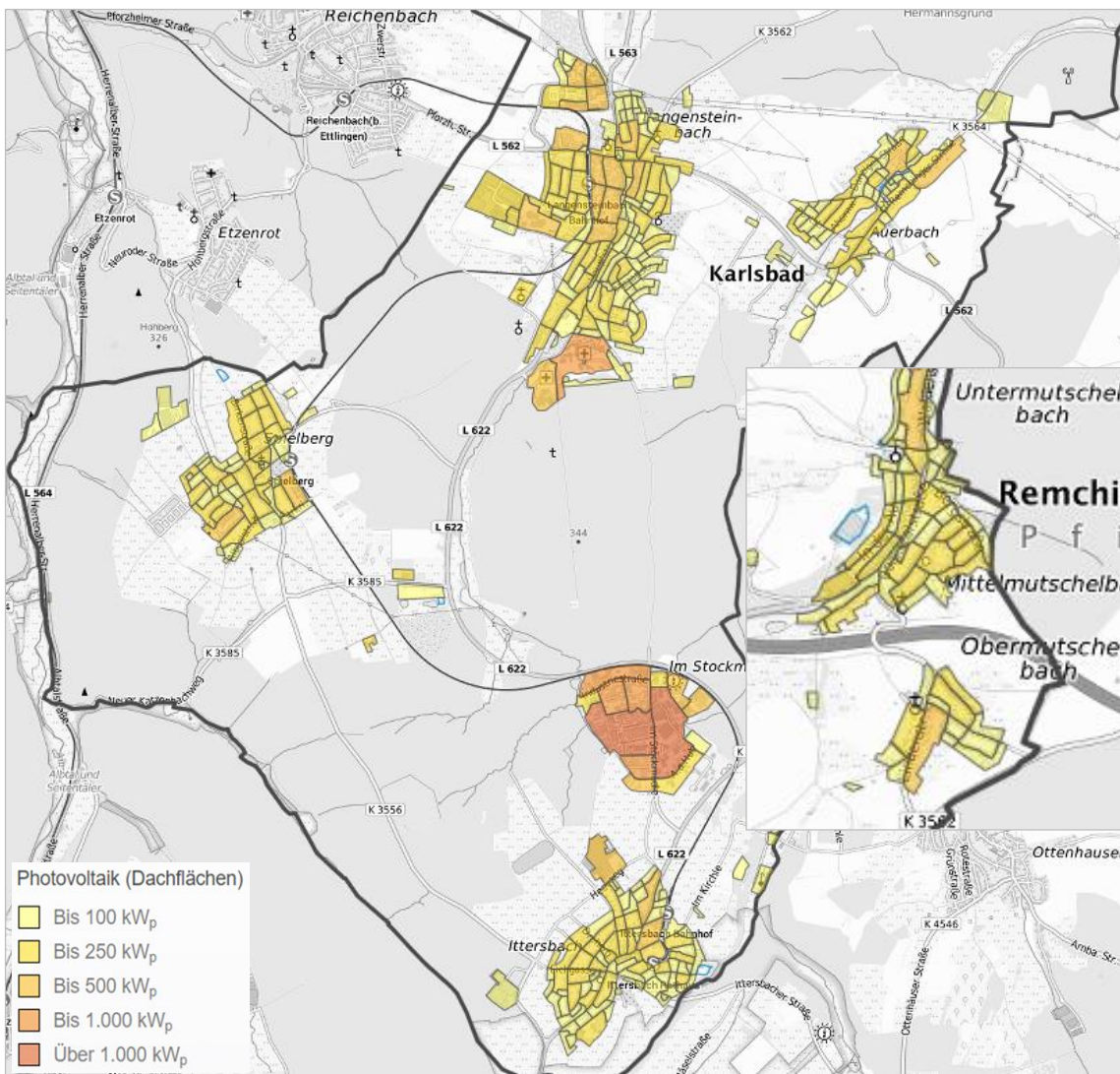
Abbildung 19: Räumliche Verortung der Dachflächenpotenziale zur Ausnutzung der Solarenergie
